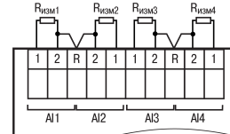
Рисунок 9 – Подключение резистивных датчиков
