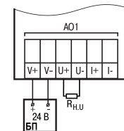
Рисунок 11 – Схема подключения к АО ПРМ-х.3 нагрузки типа У
