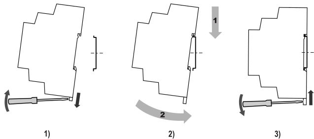
Рисунок 1 – Установка прибора
