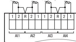
Рисунок 6 – Подключение ТС к AI ПРМ-х.3
