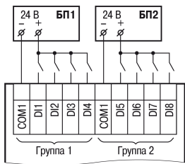
Рисунок 8 – Подключение к дискретным входам датчиков типа «сухой контакт» для сигналов 24 В
