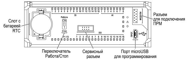
Рисунок 16 – Лицевая панель под крышкой
