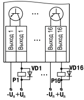
Рисунок 9 – Схема подключения нагрузок к ВЭ типа «К»
