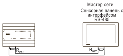
Рисунок 12 – Типовая схема подключения в режиме Slave
