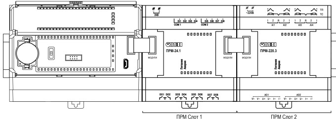
Рисунок 14 – Расположение модулей расширения на шине
