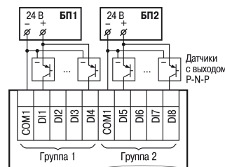
Рисунок 7 – Схема подключения к дискретным входам трехпроводных дискретных датчиков, имеющих выходной транзистор p-n-p-типа с открытым коллектором для сигналов 24 В
