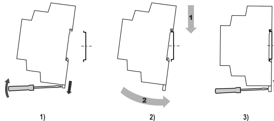
Рисунок 1 – Монтаж прибора
