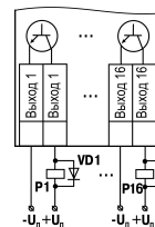
Рисунок 4 – Схема подключения нагрузок к ВЭ типа «К»
