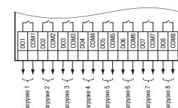
Рисунок 4 – Схема подключения нагрузок к ВЭ типа «Р»
