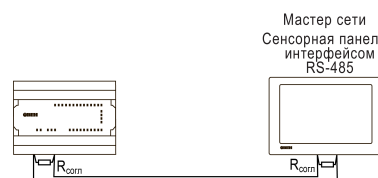
Рисунок 5 – Типовая схема подключения в режиме Slave
