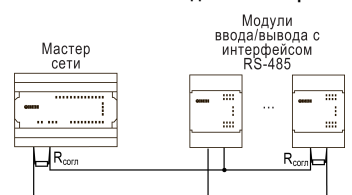
Рисунок 6 – Типовая схема подключения в режиме Master
