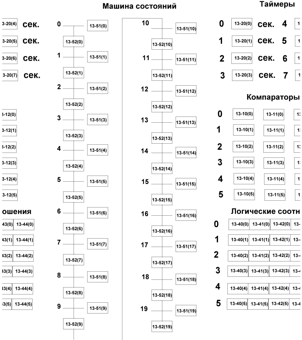
Рисунок 7.7 - Встроенный ПЛК ПЧВЗ
