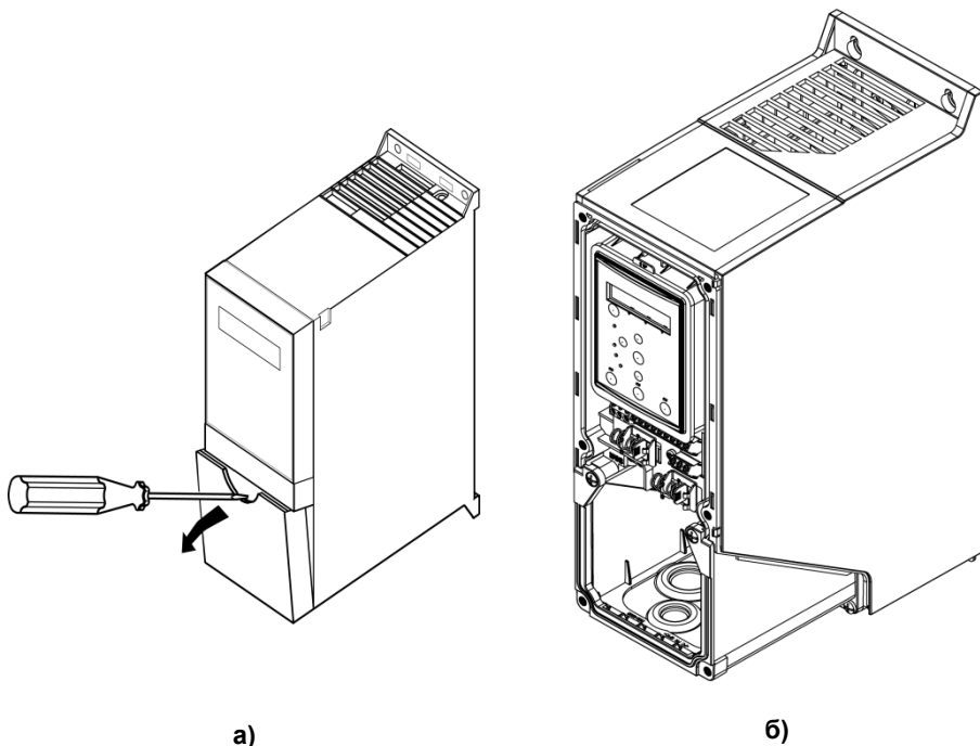
Рисунок 3.3 – Клеммный отсек: а) исполнения IP20, б) исполнения IP54
