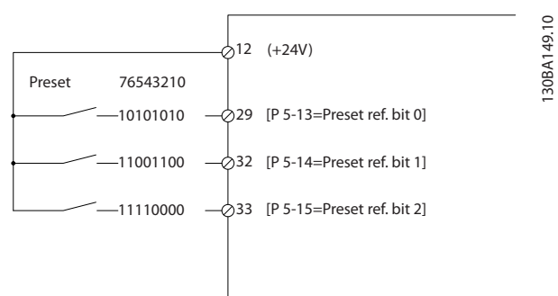
Рисунок 3.14 Схема предустановленного задания
