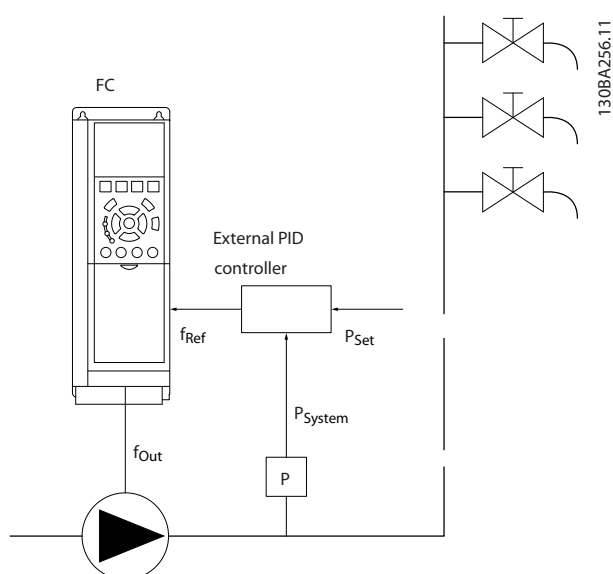
Рисунок 3.56 Система с обратной связью по давлению
