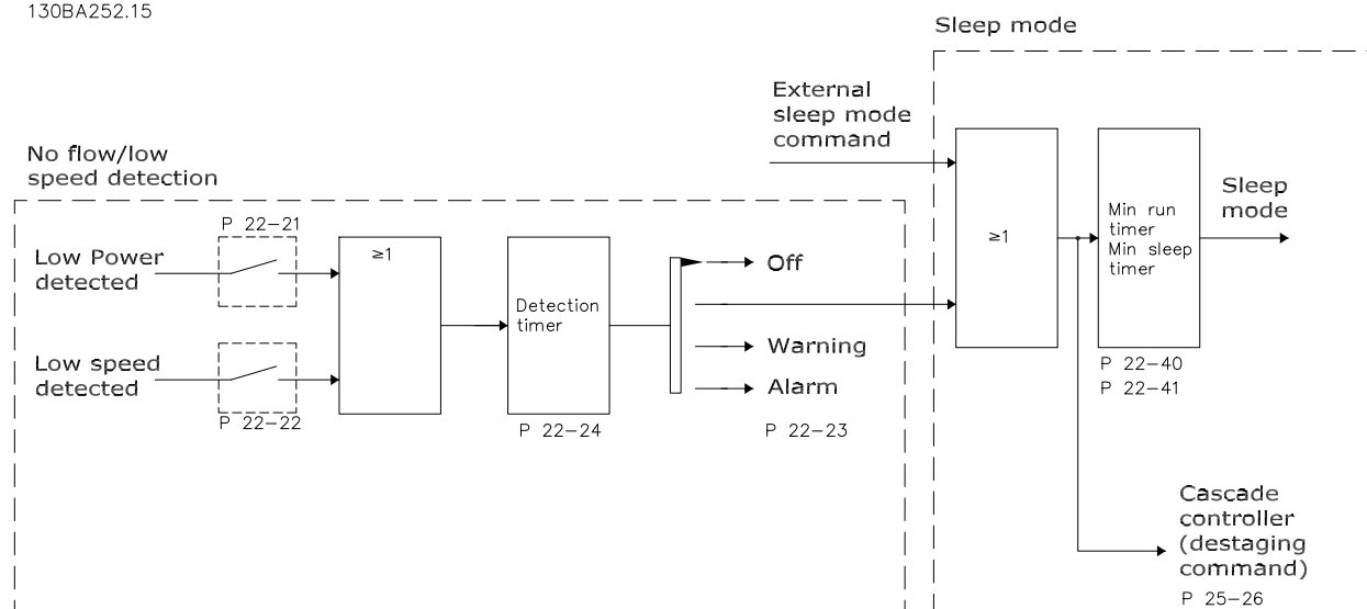
Рисунок 3.51 Схема потока сигналов
