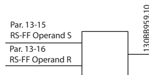
Рисунок 3.37 Триггеры сброса/установки
