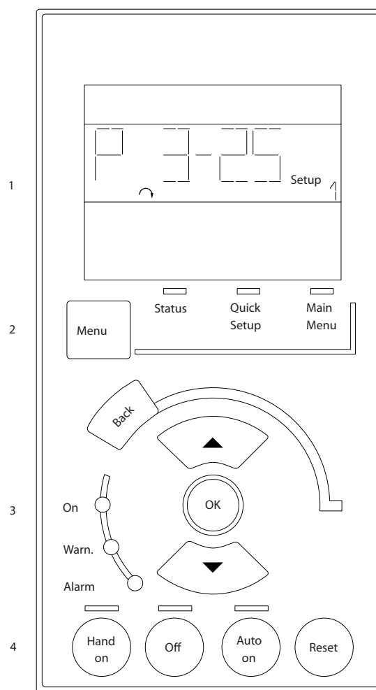
Рисунок 2.22 Кнопки LCP
