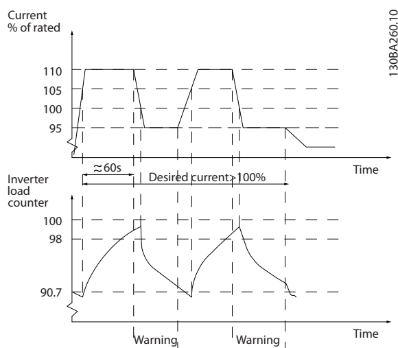
Рисунок 3.45 Выходной ток в условиях перегрузки
