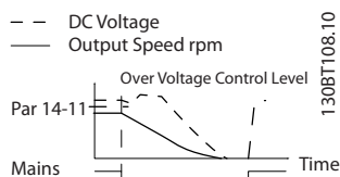
Рисунок 3.41 Управляемое замедление, более длительное замыкание цепи. Замедление длится до тех пор, пока в системе остается энергия, после этого двигатель останавливается выбегом.
