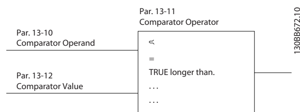
Рисунок 3.36 Компараторы
