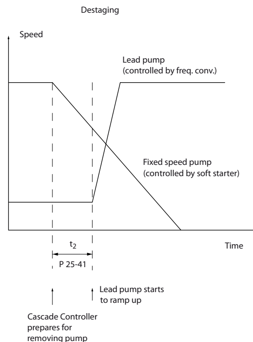
Рисунок 3.77 Выключение
