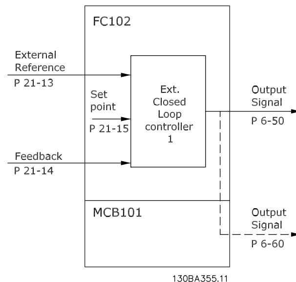
Рисунок 3.50 Расшир. CL 1, задан./обр.связь
