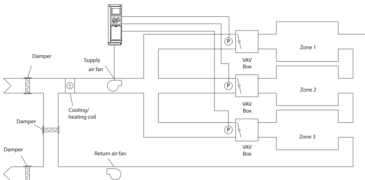
Рисунок 3.49 Схема многозонной системы
