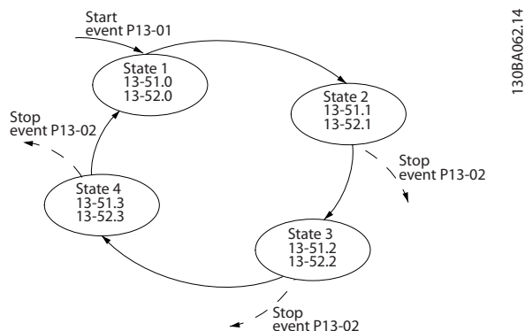
Рисунок 3.35 Действия событий интеллектуальной логики
