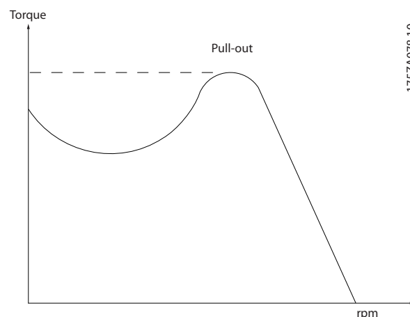
Рисунок 1.1 Момент опрокидывания
