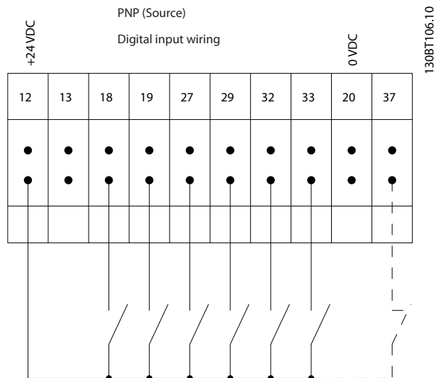
Рисунок 1.3 PNP (источник)
