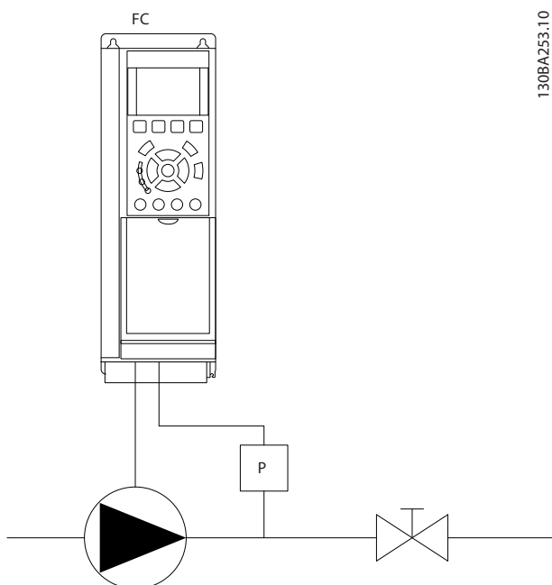
Рисунок 3.52 Схема обнаружения отсутствия потока
