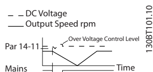
Рисунок 3.40 Управляемое замедление — короткое замыкание сети. После замедления и остановки следует разгон до заданного значения.
