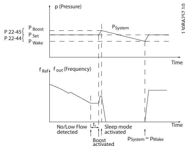
Рисунок 3.55 Система подкачки с обратной связью по давлению
