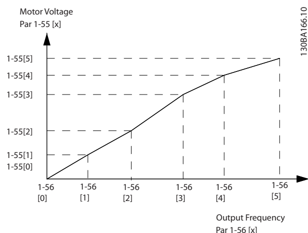
Рисунок 3.9 Характеристика U/f
