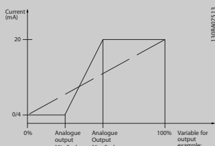
Рисунок 3.31 Зависимость выходного тока от переменной-задания
