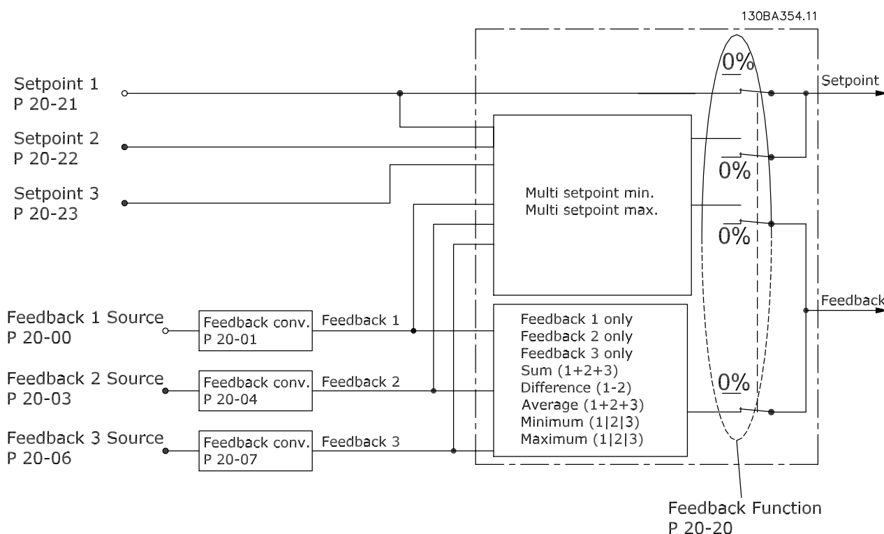
Рисунок 3.48 Входные сигналы в ПИД-регуляторе с замкнутым контуром регулирования
