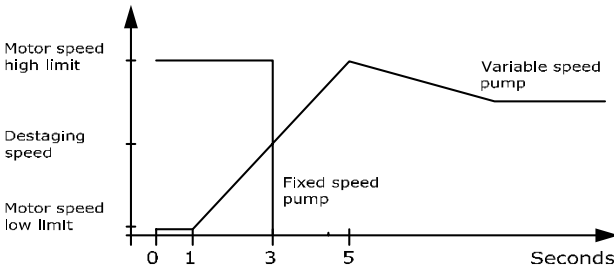
Рисунок 3.79 Порог выключения
