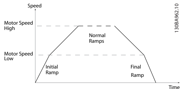
Рисунок 3.19 Время начального и конечного изменения скорости
