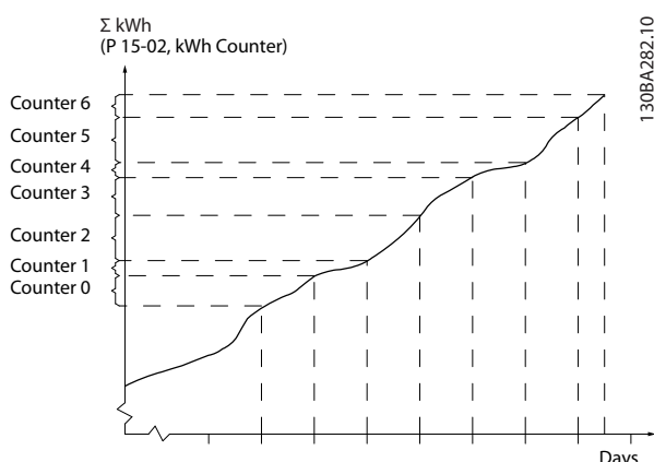
Рисунок 3.63 График энергопотребления
