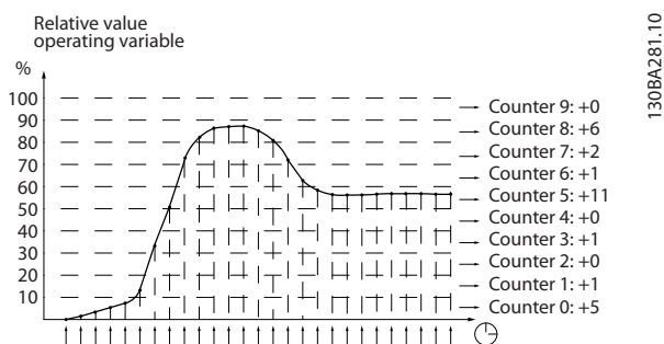
Рисунок 3.65 Время и относительные значения
