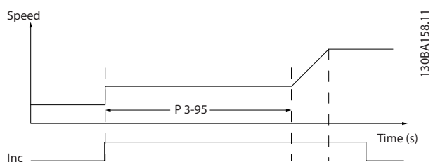
Рисунок 3.21 Задержка изменения скорости, случай 1
