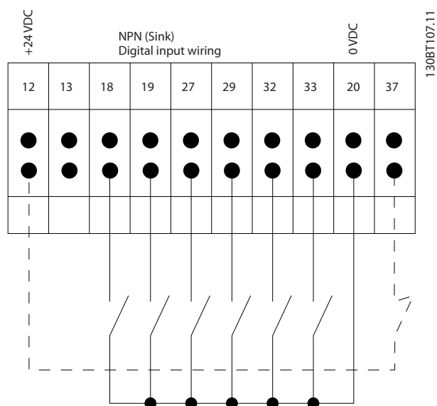
Рисунок 1.4 NPN (сток)
