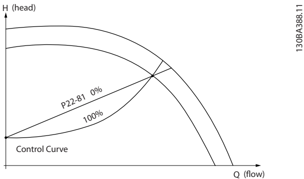
Рисунок 3.59 Квадратично-линейная аппроксимация характеристики
