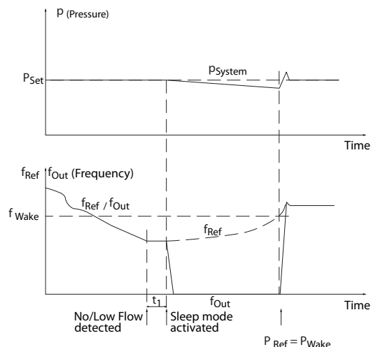
Рисунок 3.57 Система повышения давления без обратной связи по давлению
