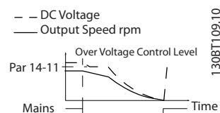
Рисунок 3.43 Кинетический резерв, более длительное замыкание сети.
