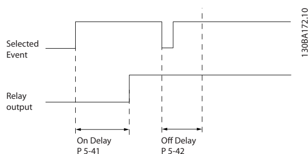
Рисунок 3.26 Задержка выключения, реле
