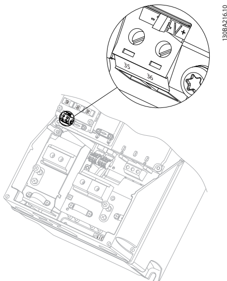
Рисунок 3.11 Подключение к резервному источнику питания 24 В (A5–C2).
