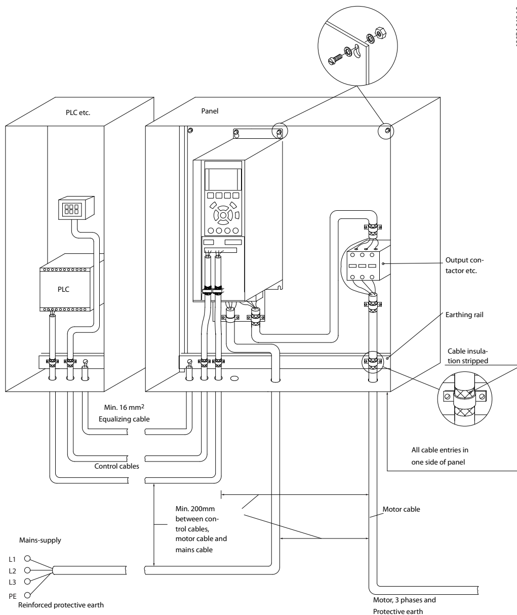
Рисунок 6.62 Корректный с точки зрения ЭМС электрический монтаж преобразователя частоты в шкафу
