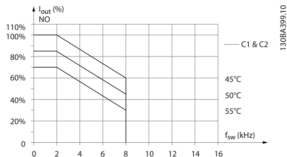
Рисунок 9.18 Снижение номинального тока I_{\text{вых.}} при различных значениях T_{\text{окр. ср., макс.}} для корпусов типа С1 и С2 для модели коммутации SFAVM в режиме нормальной перегрузки (перегрузка по крутящему моменту 110 %).
