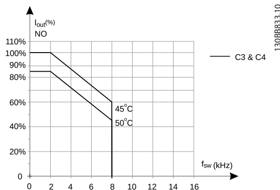
Рисунок 9.19 Снижение номинального тока I_{\text{вых.}} при различных значениях T_{\text{окр. ср., макс.}} для корпусов типа С3 и С4 для модели коммутации SFAVM в режиме нормальной перегрузки (перегрузка по крутящему моменту 110 %).
