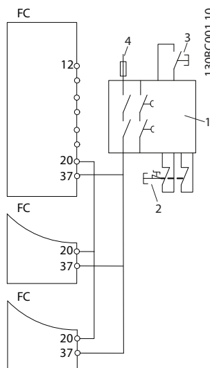
Рисунок 2.6 Пример с параллельным соединением нескольких преобразователей частоты
