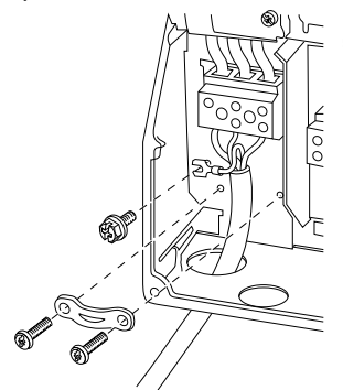
Рисунок 6.8 Подключение сети питания, корпуса типов B1 и B2 (IP 21/NEMA 1 и IP55/66/NEMA 12).
