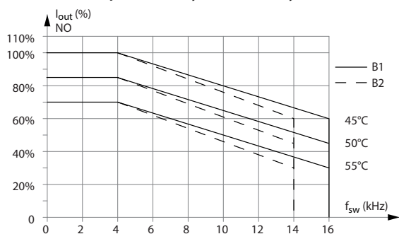
Рисунок 9.8 Снижение номинального тока I_{\text{вых.}} при различных значениях T_{\text{окр. ср. макс.}} для корпусов типа B1 и B2 для модели коммутации 60° AVM в режиме нормальной перегрузки (перегрузка по крутящему моменту 110 %).
