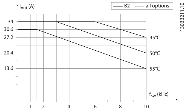
Рисунок 9.14 Снижение номинального выходного тока при частотах коммутации и окружающей температуре для типа корпуса B2 с моделью коммутации 60° AVM. Примечание. На графике показано абсолютное значение тока, действительное для высокой и нормальной перегрузки.
