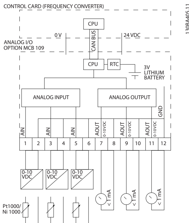
Рисунок 3.12 Принципиальная схема аналоговых входов/выходов, предусмотренных в преобразователе частоты.
