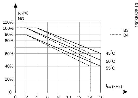
Рисунок 9.9 Снижение номинального тока I_{\text{вых.}} при различных значениях T_{\text{окр. ср. макс.}} для корпусов типа B3 и B4 для модели коммутации 60° AVM в режиме нормальной перегрузки (перегрузка по крутящему моменту 110 %).
