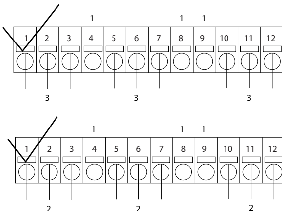
Рисунок 3.9 Подключение
