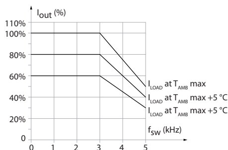
Рисунок 9.7 Снижение номинального тока I_{\text{вых.}} при различных значениях T_{\text{окр. ср. макс.}} для корпуса типа A3
