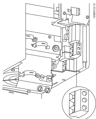
Рисунок 6.9 Подключение сети питания, корпуса типа V3 (IP20)
