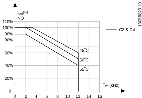
Рисунок 9.17 Снижение номинального тока I_{\text{вых.}} при различных значениях T_{\text{окр. ср., макс.}} для корпусов типа С3 и С4 для модели коммутации 600° AVM в режиме нормальной перегрузки (перегрузка по крутящему моменту 110 %).
