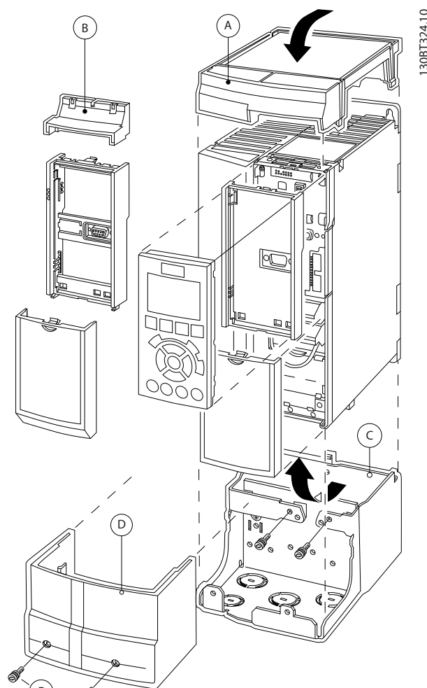
Рисунок 3.20 Тип корпуса A3
