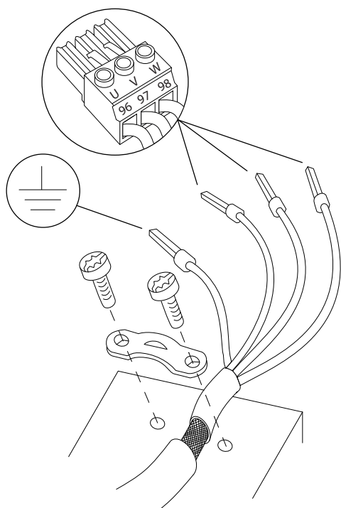
Рисунок 6.14 Подключение двигателя
