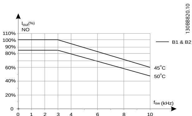
Рисунок 9.12 Снижение номинального выходного тока при частотах коммутации и окружающей температуре для преобразователей частоты на 600 В с типом корпуса B, моделью коммутации 60° AVM в режиме нормальной перегрузки
