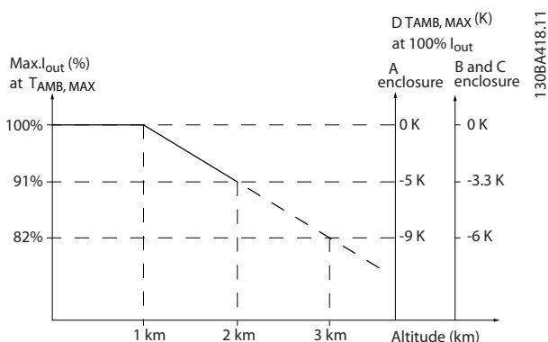
Рисунок 9.24 Снижение номинального выходного тока при максимальной температуре окружающей среды T_{окр. ср., макс.} в зависимости от высоты над уровнем моря для типов корпусов A, B и C. В случае высоты над уровнем моря более 2000 м обратитесь в Danfoss относительно требований PELV.
