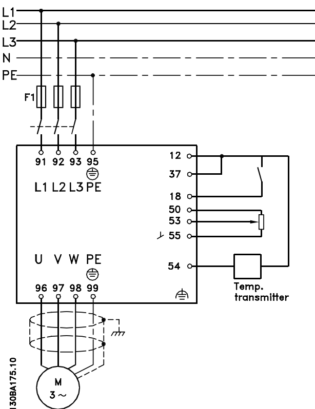
Рисунок 6.63 Схема электрического соединения
