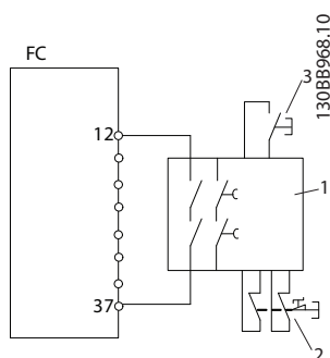
Рисунок 2.3 Пример с безопасным отключением крутящего момента (STO)
