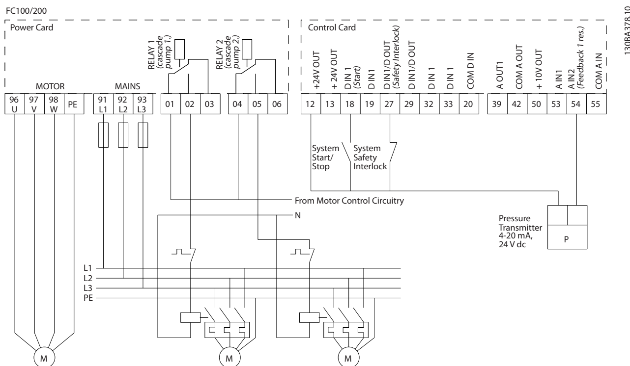
Рисунок 7.11 Схема электрических соединений каскадного контролера
