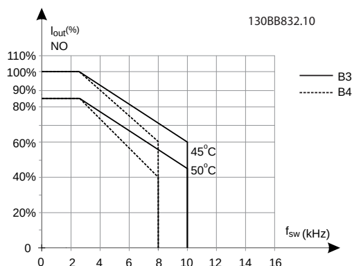
Рисунок 9.11 Снижение номинального тока I_{\text{вых.}} при различных значениях T_{\text{окр. ср. макс.}} для корпусов типа B3 и B4 для модели коммутации SFAVM в режиме нормальной перегрузки (перегрузка по крутящему моменту 110 %).
