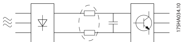
Рисунок 2.33 Токи гармоник
