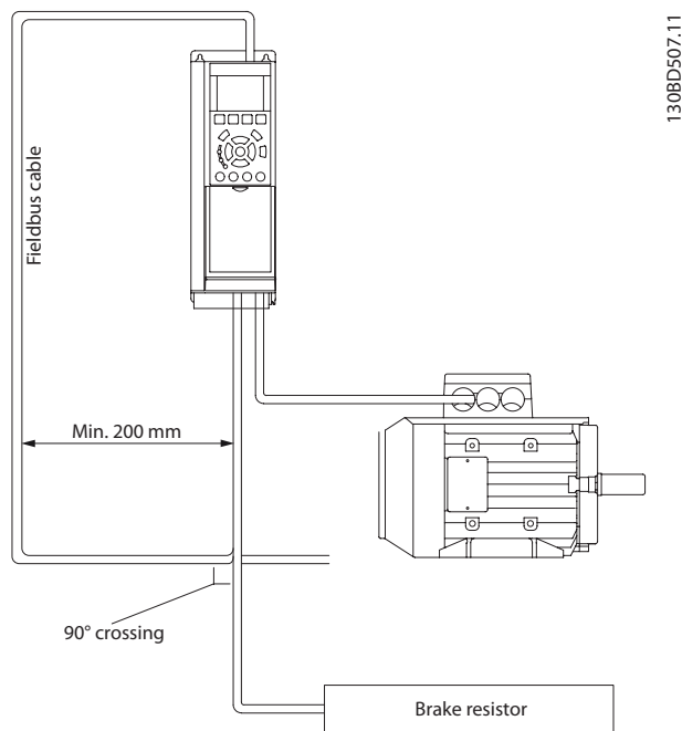
Рисунок 8.4 Прокладка кабелей
