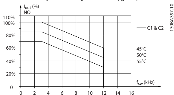
Рисунок 9.16 Снижение номинального тока I_{\text{вых.}} при различных значениях T_{\text{окр. ср., макс.}} для корпусов типа С1 и С2 для модели коммутации 60° AVM в режиме нормальной перегрузки (перегрузка по крутящему моменту 110 %).
