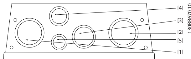
Рисунок 6.32 Отверстия с резьбовыми уплотнениями B2 — IP55
