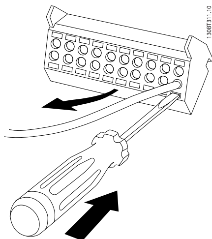
Рисунок 6.52 Вставьте кабель
