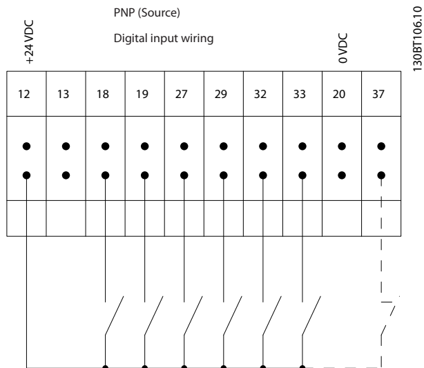
Рисунок 6.56 Входная полярность PNP (источник)
