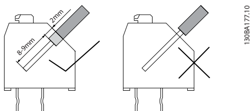
Рисунок 3.8 Установка
