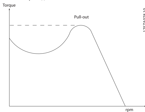
Рисунок 1.1 Момент опрокидывания
