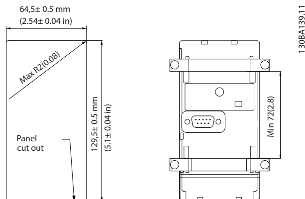
Рисунок 3.18 Размеры
