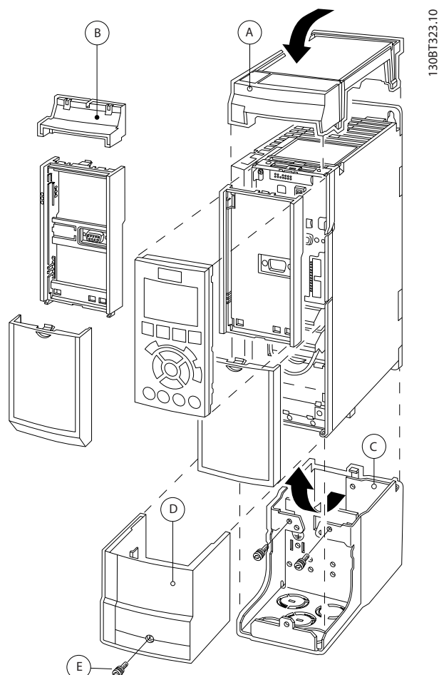
Рисунок 3.19 Тип корпуса A2
