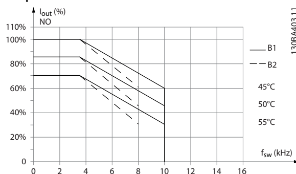
Рисунок 9.10 Снижение номинального тока I_{\text{вых.}} при различных значениях T_{\text{окр. ср. макс.}} для корпусов типа B1 и B2 для модели коммутации SFAVM в режиме нормальной перегрузки (перегрузка по крутящему моменту 110 %).
