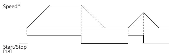
Рисунок 7.1 Клемма 37: Предусматривается только с функцией безопасного останова!
