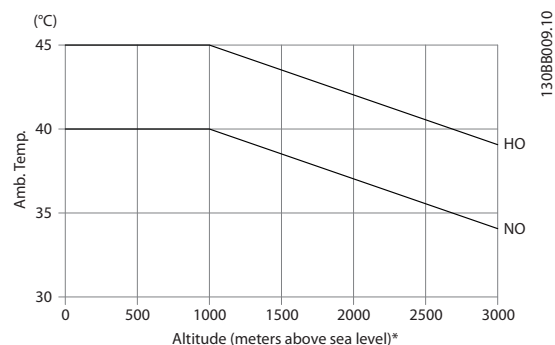
Рисунок 9.26 Пример: При высоте 2000 м и температуре 45 °C ( T_{окр.ср., макс.} - 3,3 K) доступное значение выходного тока составляет 91 % от номинального значения. При температуре 41,7 °C доступное значение выходного тока составляет 100 % от номинального.
