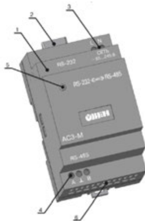
Рисунок 4.1 – Внешний вид прибора AC3-M
